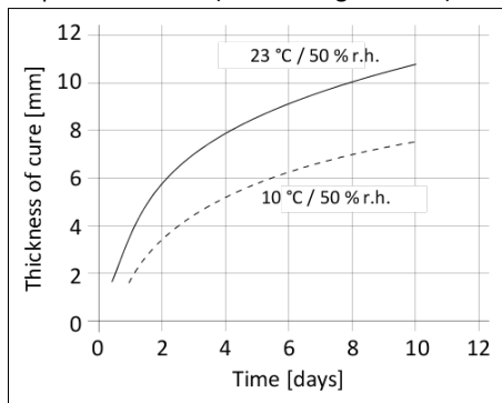
Diagramma 1: Velocità di indurimento per Sikaflex®-291i
