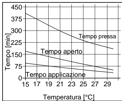
Diagramma 1: Tempo aperto, tempo di pressa e tempo di applicazione per SikaForce®-7720 L105
