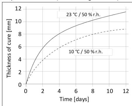
Diagramma 1: Velocità di indurimento per Sikaflex®-212 FC
