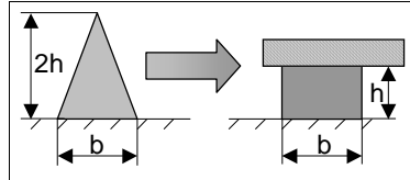
Figura 1: Configurazione raccomandata del cordolo
